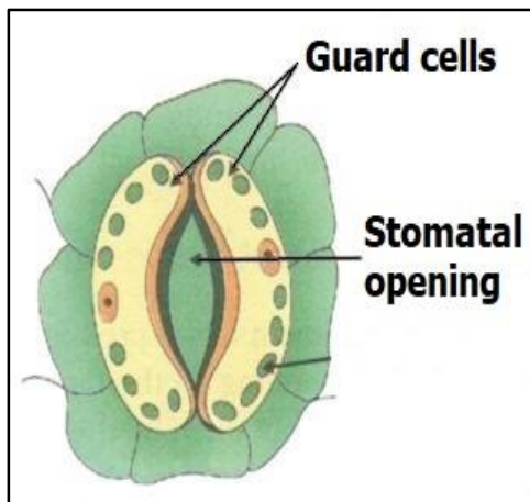
a) Stomata
